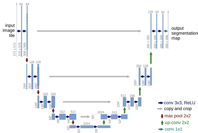
Fig. 1. Arquitectura U-Net introducida en [2]
